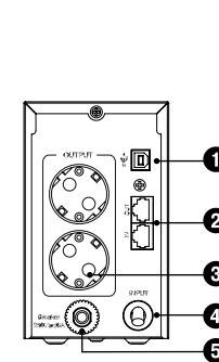
Задняя панель моделей с евророзетками
