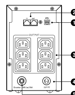
Задняя панель моделей с розетками IEC C13
