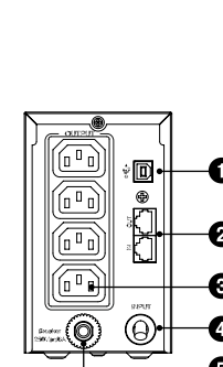
Задняя панель моделей с розетками IEC C13
