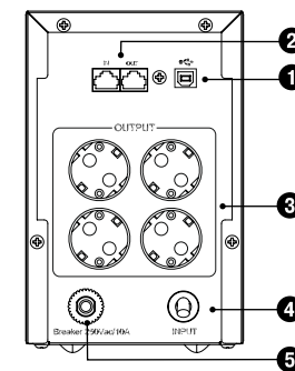
Задняя панель моделей с евророзетками
